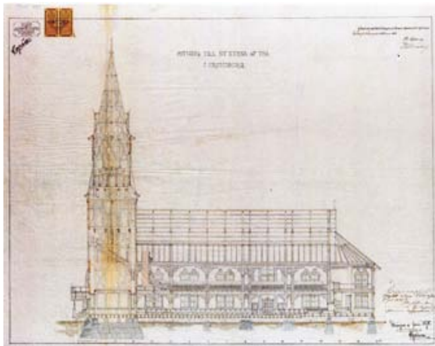
Ritning till ny kyrka af trä i Kronoborg, F.A. Sjöström 1875.
