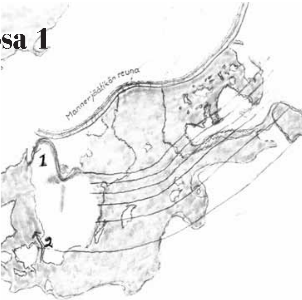
Tässä piirroksessa harmaana näkyy Ancylus-järven laajuus (rannansiirtymisen) maksimin aikana. Lasku-uoma maksimin aikana (1) ja sen jälkeen (2). Keskellä piirrosta Itämeri, oikealla ylhäällä Etelä- ja Keski-Suomi.
